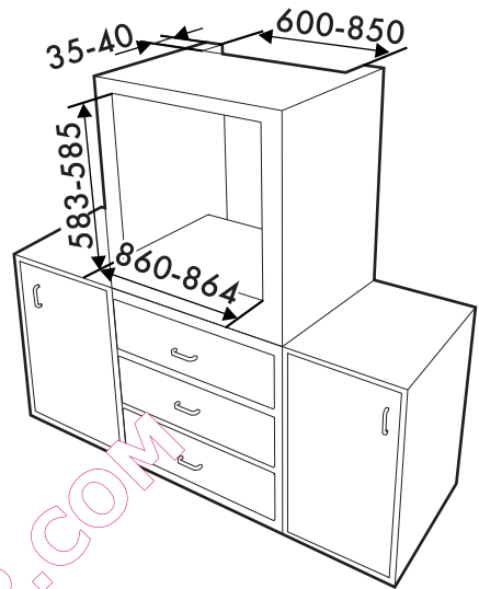
Encastrement en colonne (mm)
