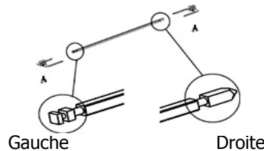
3. Retirer les fourches du tournebroche
